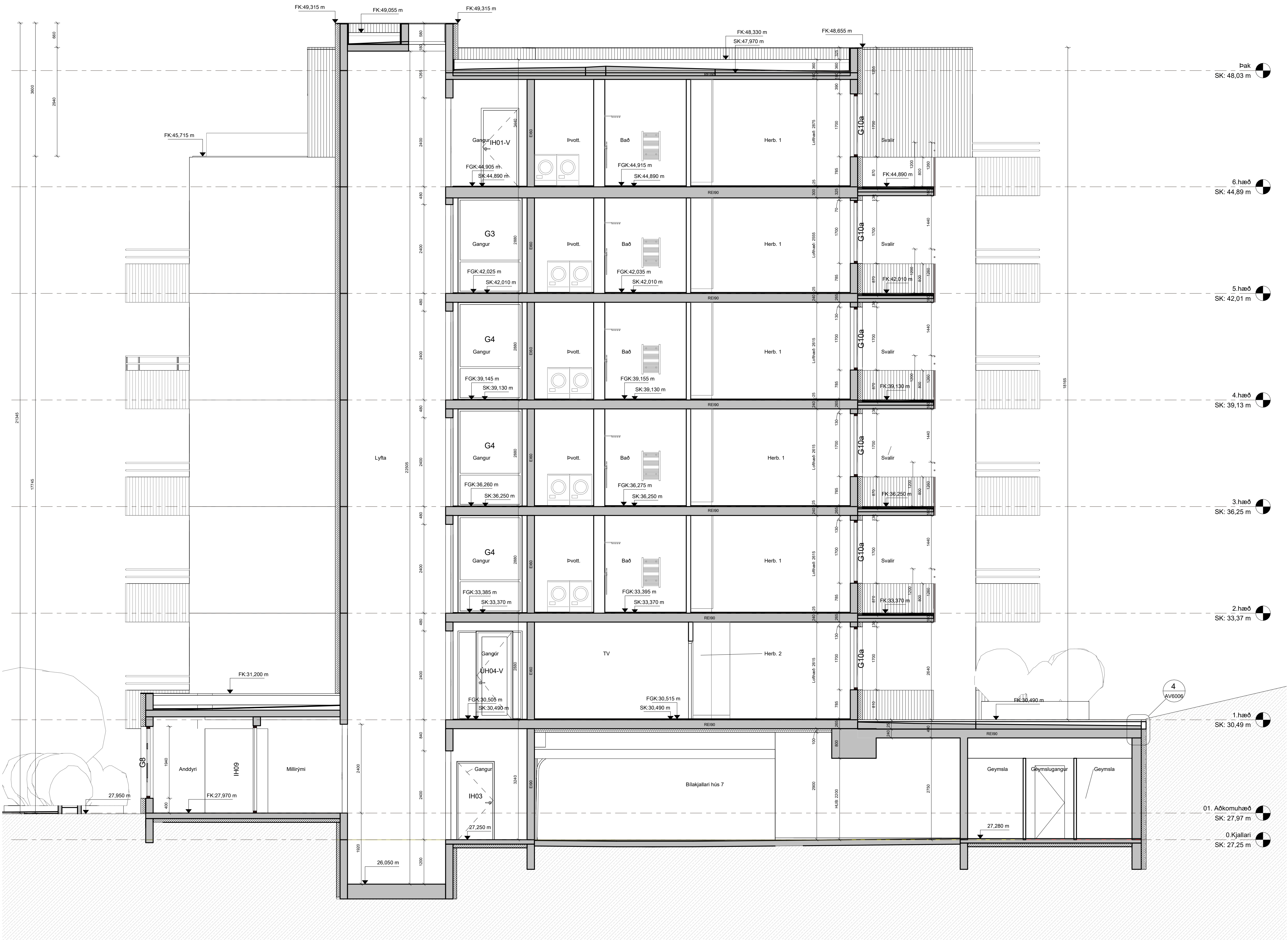
F-F. mkv: 1 : 50
